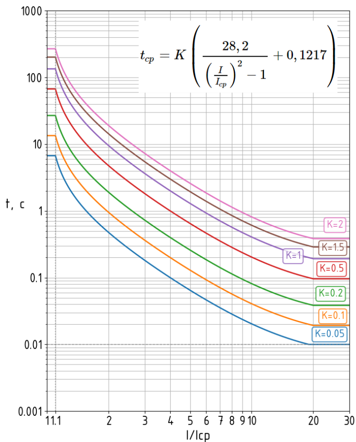
Рисунок И.6 – Кривая F (Чрезвычайно инверсная ANSI)
