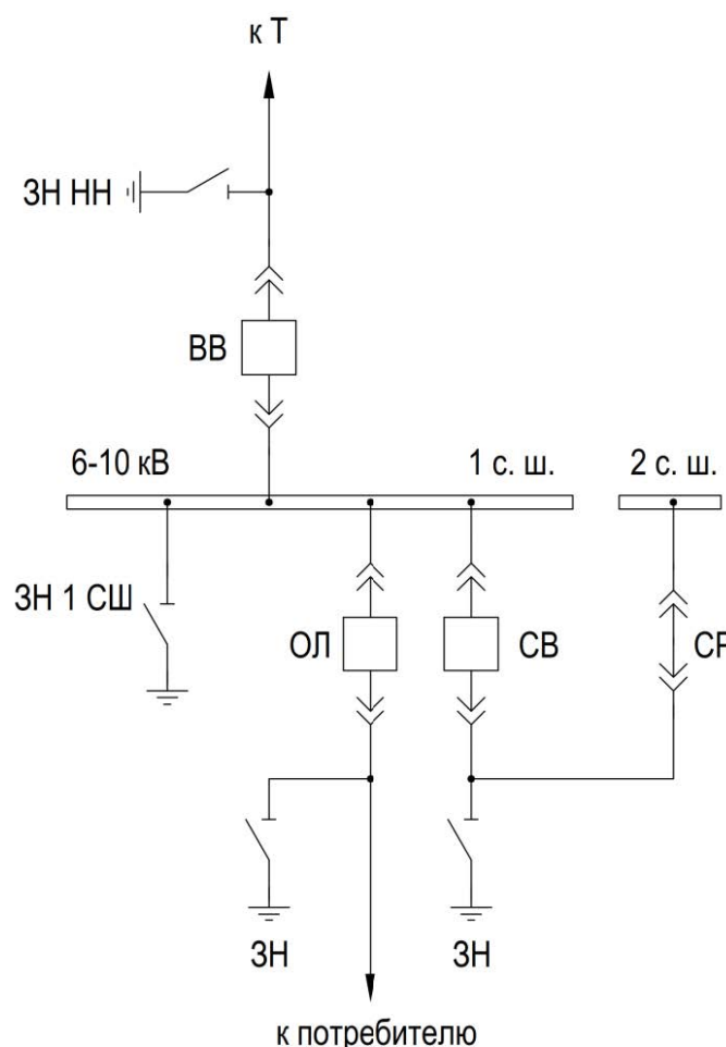
Рисунок 2.58 – Поясняющая схема первичной сети для алгоритмов оперативной блокировки КА
