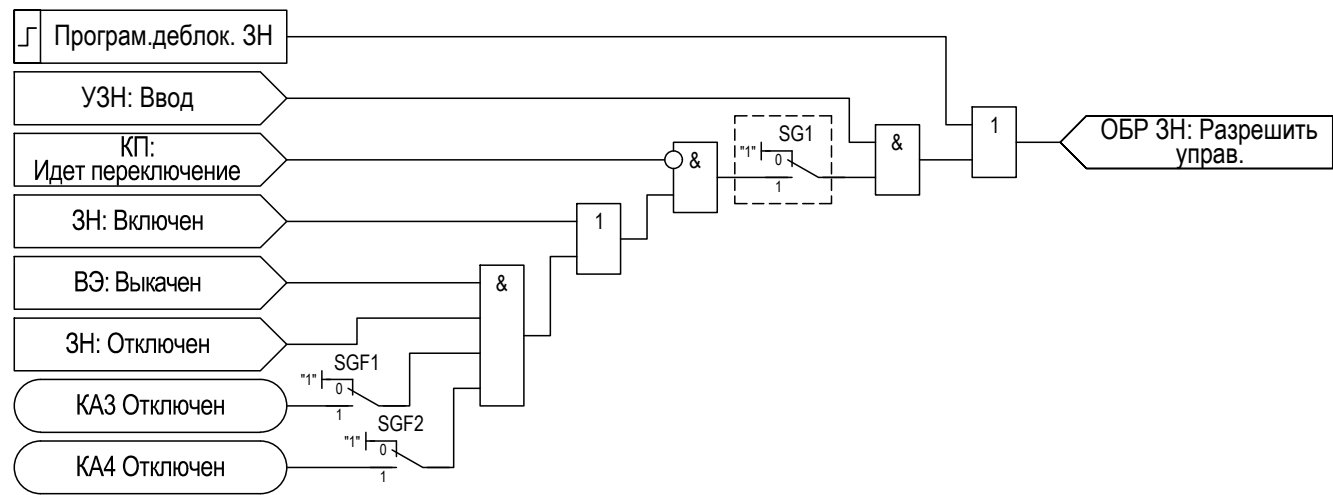
Рисунок 2.61 – Функциональная схема «ОБР 3Н»
