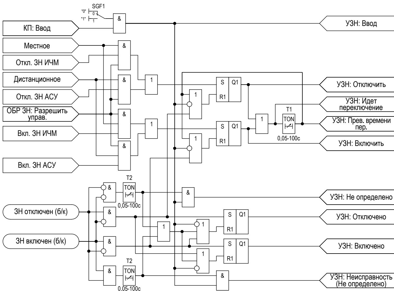
Рисунок 2.57 – Функциональная схема «УЗН»
